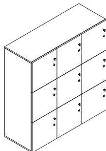
Locker LK45C 3x3 L: 135, W: 50, H: 145 cm
