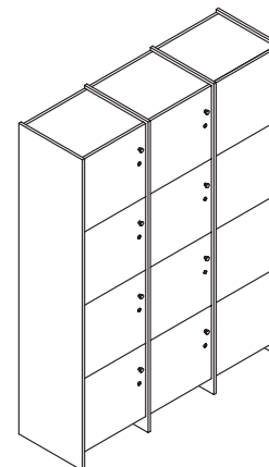
Locker LK54C 3x4 L: 158, W: 50, H: 210 cm
